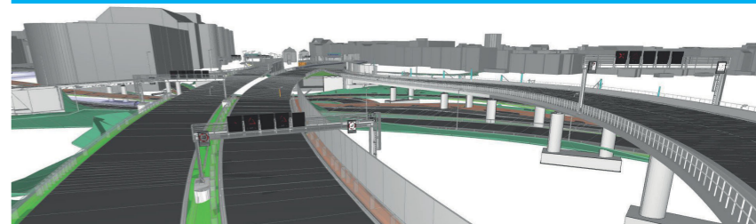
BIM-Modell Autobahndreieck Funkturm (Berlin)
